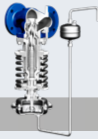
自力式控制阀 PREDU® / PREDEX® / PRESO® / TEMPROL®
